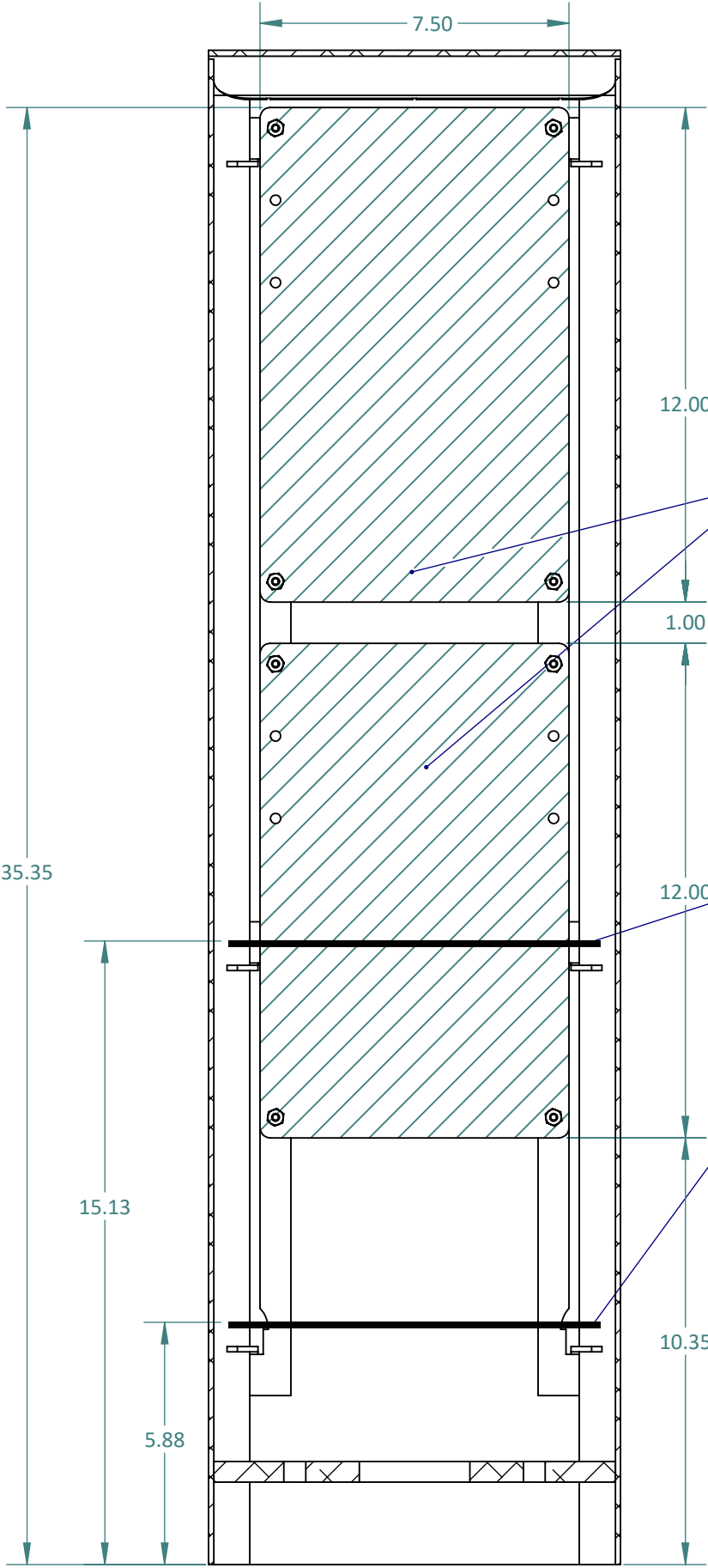
SECTION B-B SCALE 1 : 4
