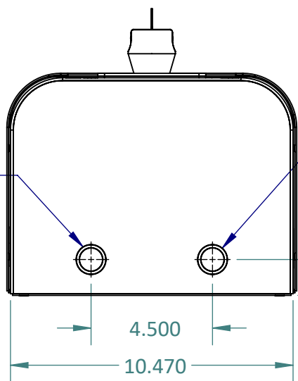
KNOCKOUT FOR 0.75" CONDUIT
